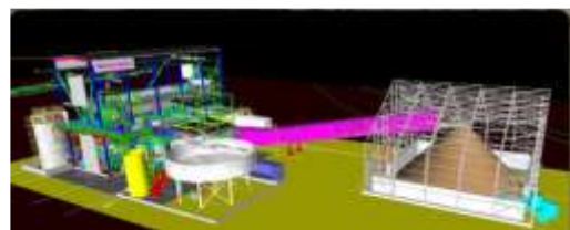
Постројка за подготовка на јаловина за суво одлагање
